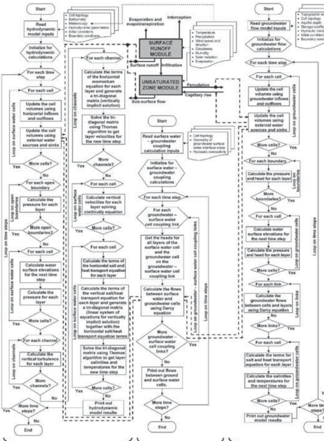
Kavramsal hidrolojik model kurgusu
