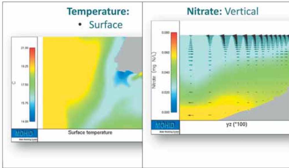
Şekil 2 Bir deniz deşarjı modelinde GKA ile elde edilen sıcaklık ve nitrat dağılımı
