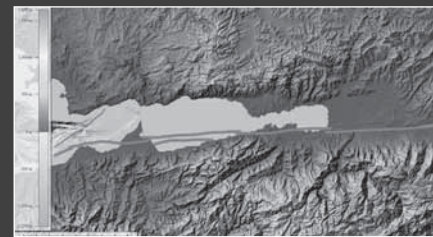
17 Ağustos 1999'da kırılan fay hattı
